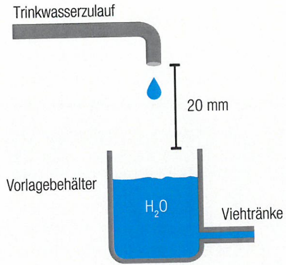
Abb. 2: Schematische Darstellung des freien Auslaufs mit Vorlagebehälter; der freie Abstand von mindestens 20 mm darf nicht unterschritten werden.
